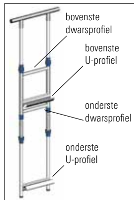
Afbeelding 16: Details Veiligheidskopleuning
